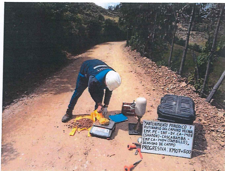
FIGURA N° 31. Ensayo de Densidad de Suelo en Campo. Progresiva 07 + 500 (Método del cono de arena).
