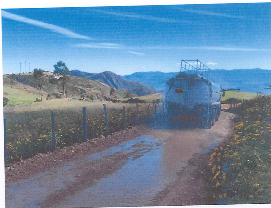
SE OBSERVA LA VERIFICACION DEL REGADO DE LA CAPA DE AFIRMADO CON CAMION CISTERNA CON UNA CAPACIDAD DE 5,000 GALONES.
