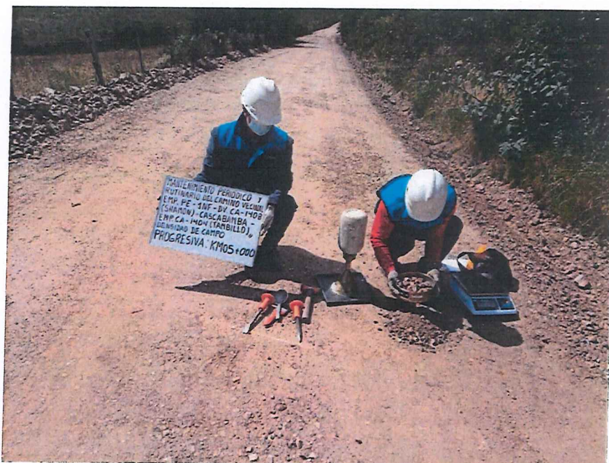
FIGURA N° 21. Ensayo de Densidad de Suelo en Campo. Progresiva 05 + 000 (Método del cono de arena).
