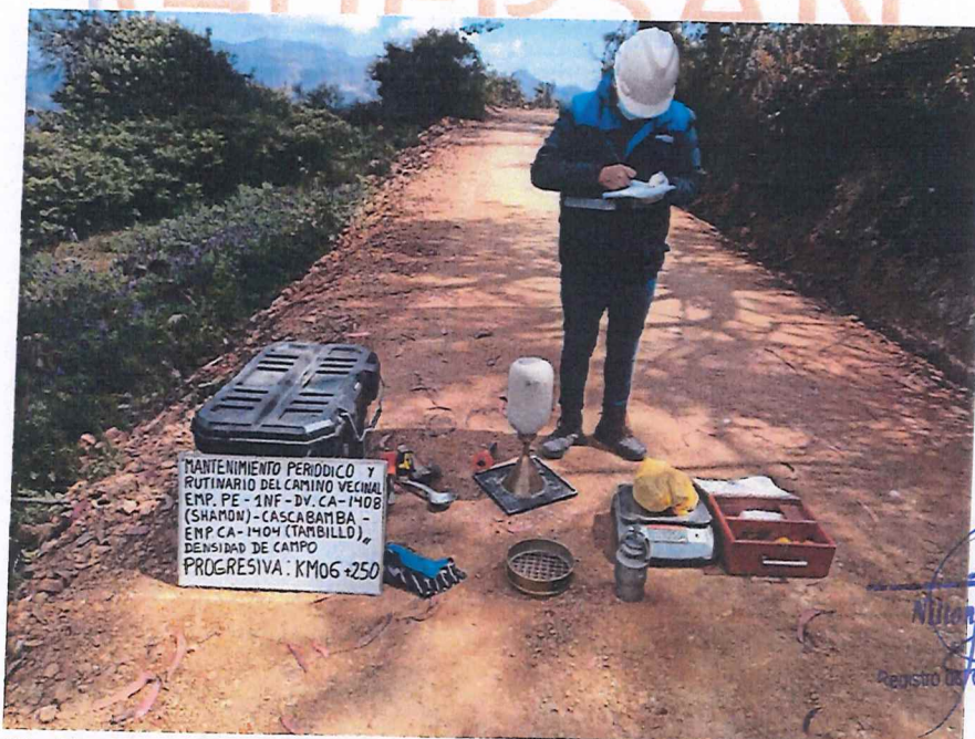
FIGURA N° 26. Ensayo de Densidad de Suelo en Campo. Progresiva 06 + 250 (Método del cono de arena).
