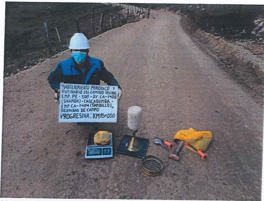
FIGURA N° 61. Ensayo de Densidad de Suelo en Campo. Progresiva 15 + 000 (Método del cono de arena).
