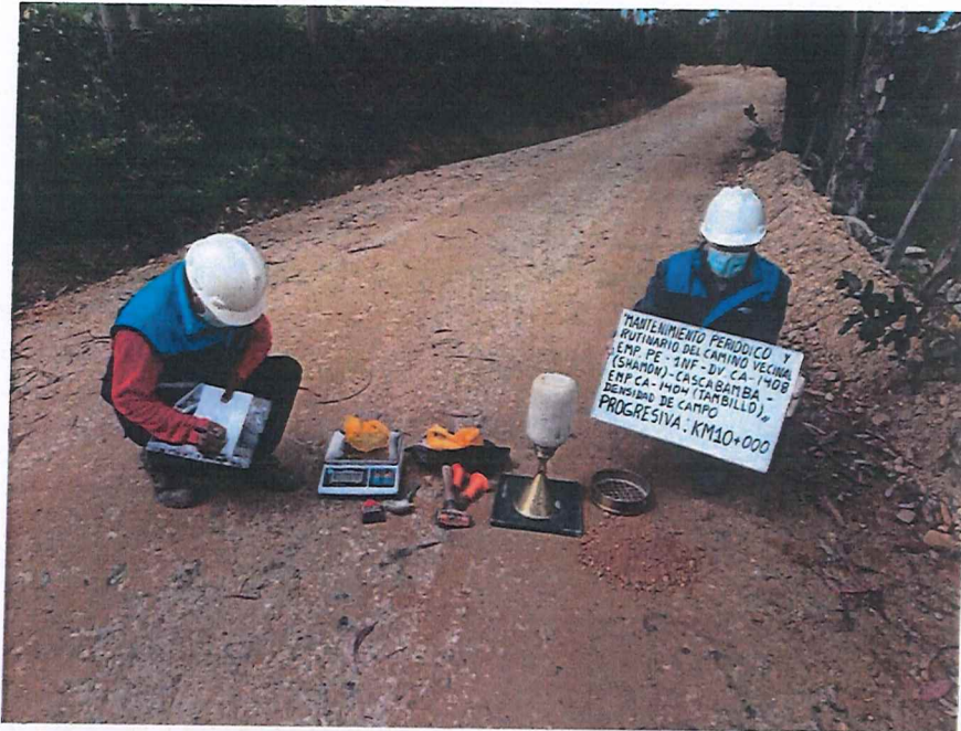
FIGURA N° 41. Ensayo de Densidad de Suelo en Campo. Progresiva 10 + 000 (Método del cono de arena).
