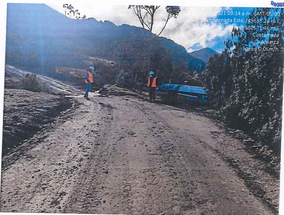
Fotografía 46. Culminación del refine y compactación de material granular para afirmado e=0.15m
