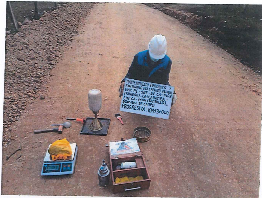
FIGURA N° 53. Ensayo de Densidad de Suelo en Campo. Progresiva 13 + 000 (Método del cono de arena).
