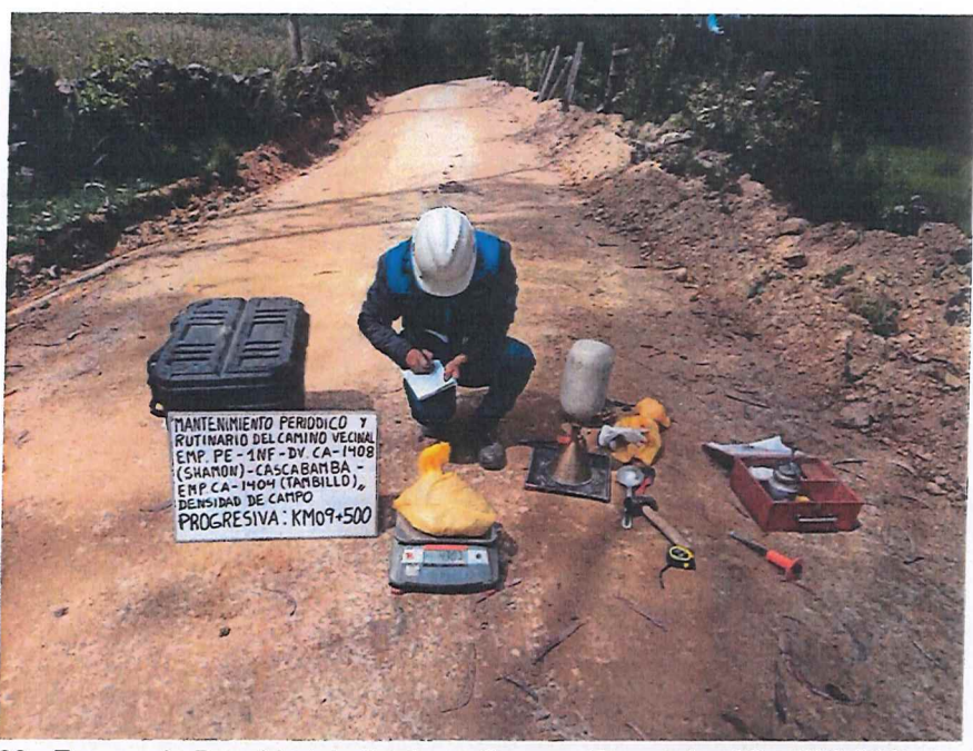
FIGURA N° 39. Ensayo de Densidad de Suelo en Campo. Progresiva 09 + 500 (Método del cono de arena).
