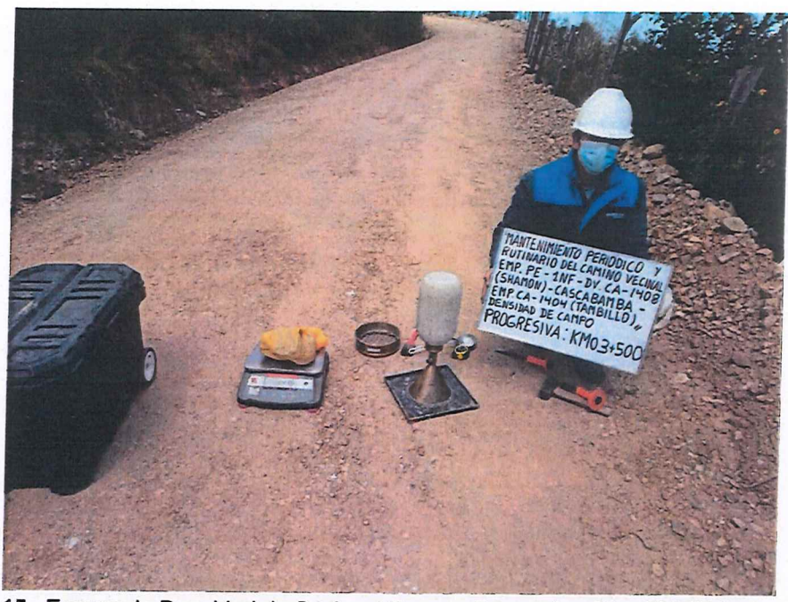
FIGURA N° 15. Ensayo de Densidad de Suelo en Campo. Progresiva 03 + 500 (Método del cono de arena).
