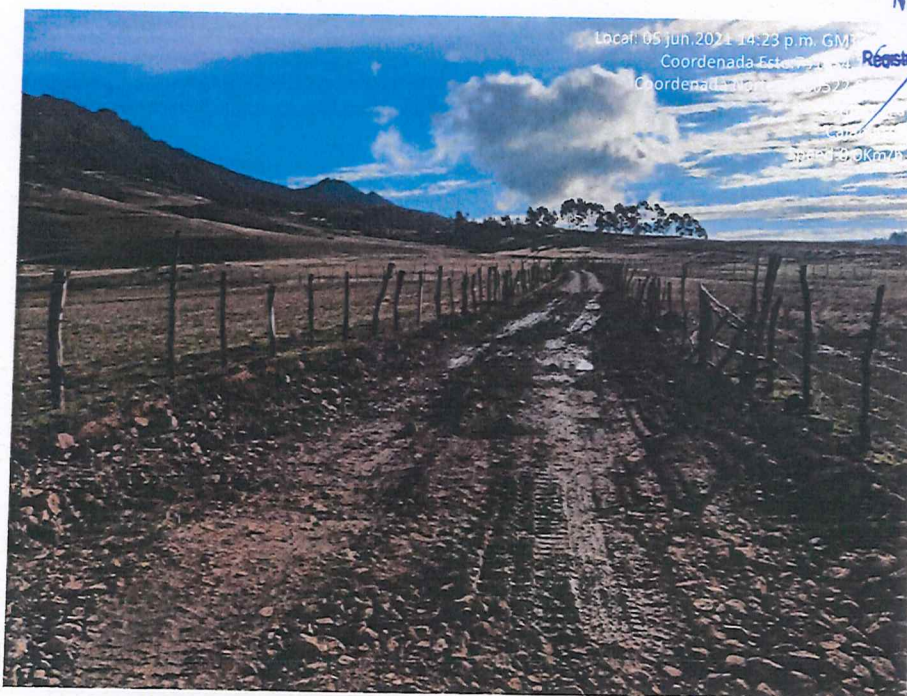
Fotografía 28. Mejoramiento de la capa nivelante con material grueso para mejorar drenaje.
