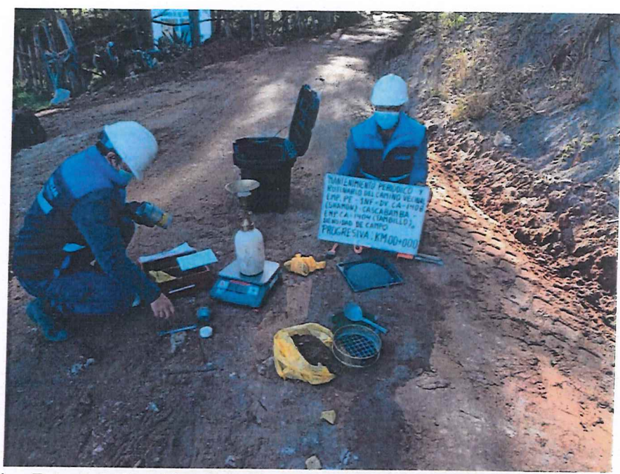
FIGURA N° 1. Ensayo de Densidad de Suelo en Campo. Progresiva 00 + 000 (Método del cono de arena).
