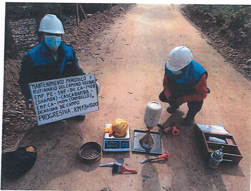
FIGURA N° 55. Ensayo de Densidad de Suelo en Campo. Progresiva 13 + 500 (Método del cono de arena).
