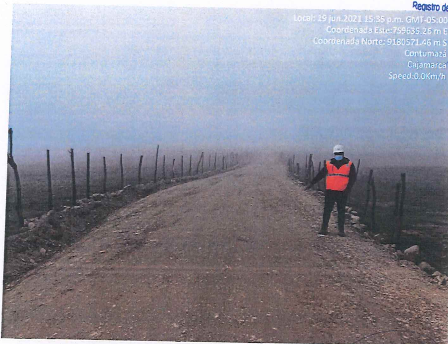
Fotografía 56. Resultado de la compactación del afirmado con bombeo del 3%.
