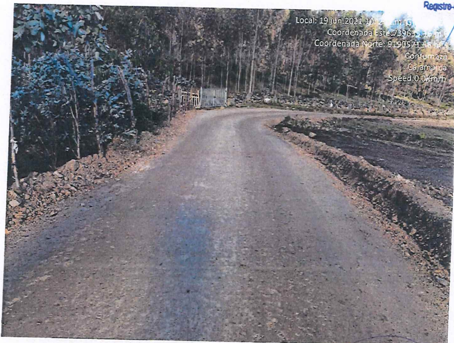
Fotografía 48. Resultado de la compactación del afirmado.
