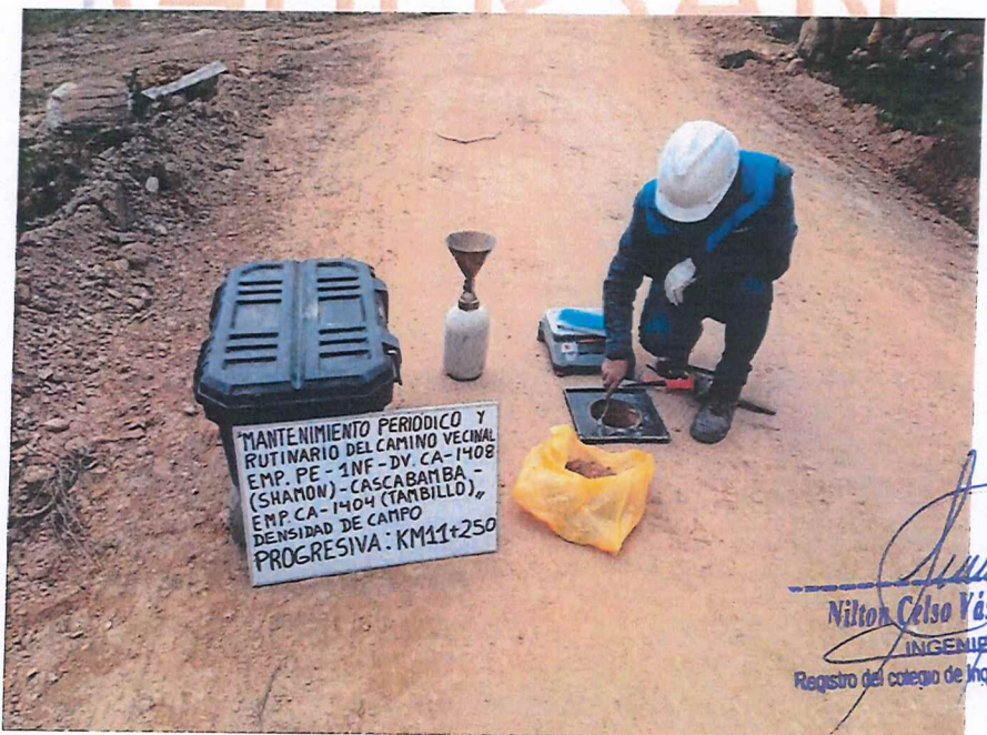
FIGURA N° 46. Ensayo de Densidad de Suelo en Campo. Progresiva 11 + 250 (Método del cono de arena).
