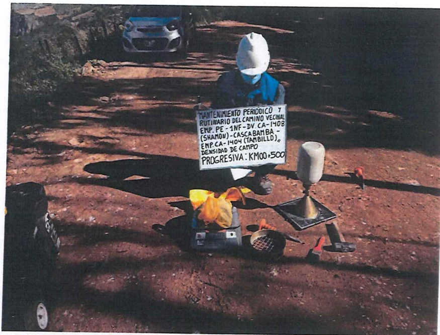
FIGURA N° 3. Ensayo de Densidad de Suelo en Campo. Progresiva 00 + 500 (Método del cono de arena).
