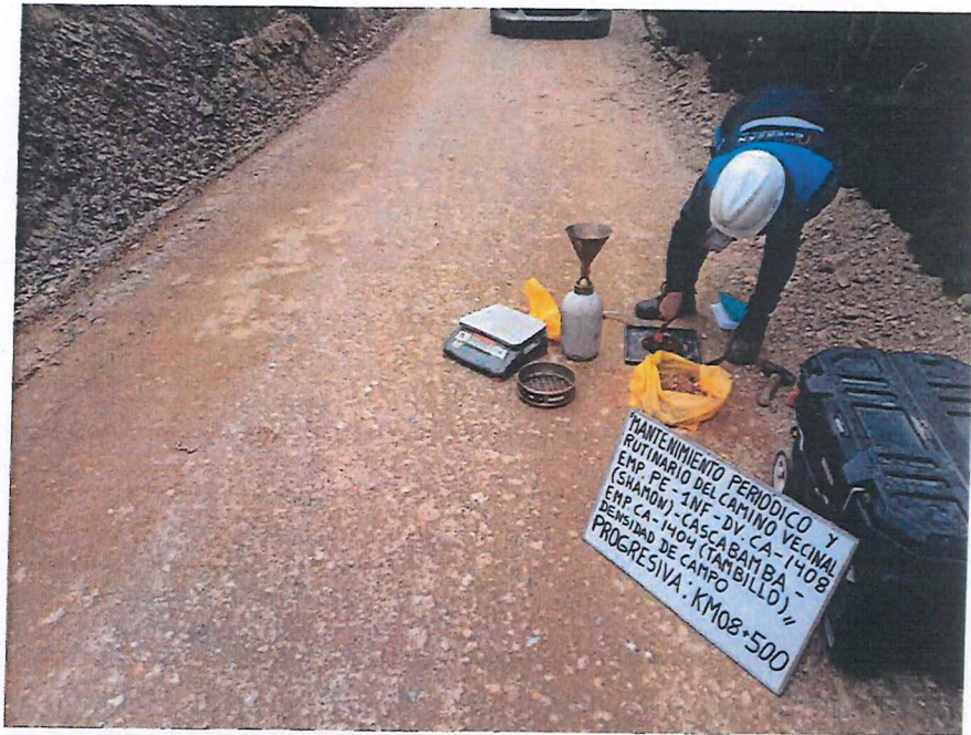
FIGURA N° 35. Ensayo de Densidad de Suelo en Campo. Progresiva 08 + 500 (Método del cono de arena).
