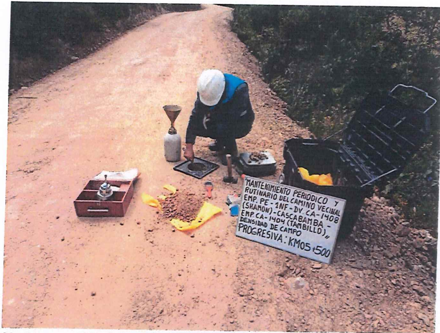
FIGURA N° 23. Ensayo de Densidad de Suelo en Campo. Progresiva 05 + 500 (Método del cono de arena)
