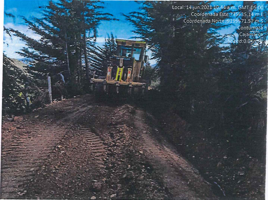
Fotografía 35. Conformación y reconformación de cunetas.
