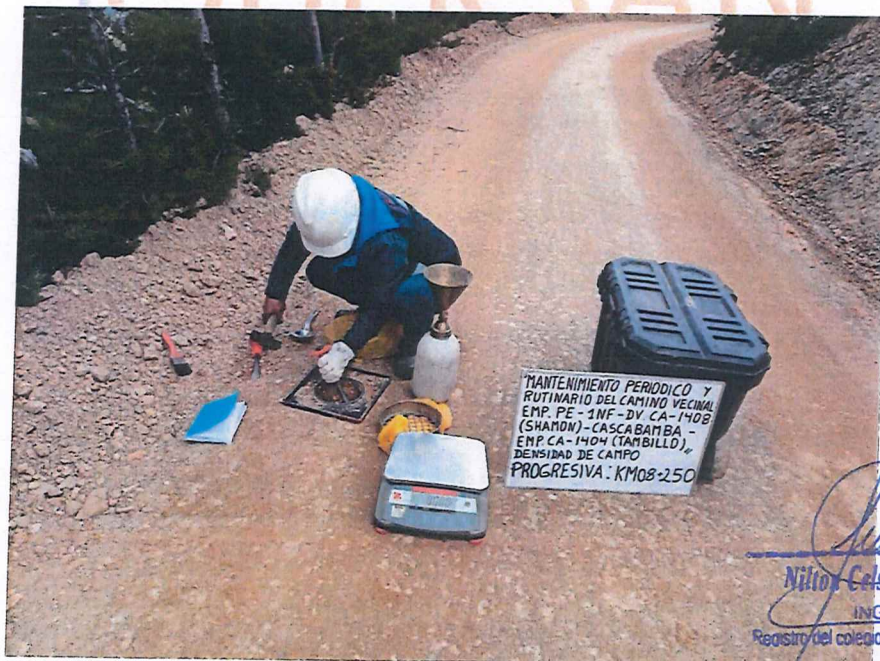
FIGURA N° 34. Ensayo de Densidad de Suelo en Campo. Progresiva 08 + 250 (Método del cono de arena).
