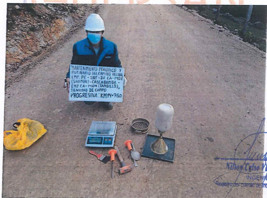
FIGURA N° 60. Ensayo de Densidad de Suelo en Campo. Progresiva 14 + 750 (Método del cono de arena).
