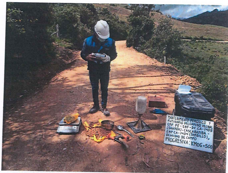
FIGURA N° 27. Ensayo de Densidad de Suelo en Campo. Progresiva 06 + 500 (Método del cono de arena).
