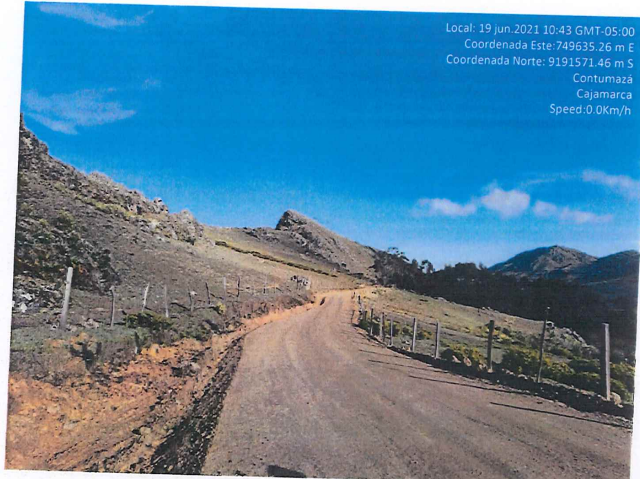
Fotografía 49. Resultado de la compactación del afirmado.
