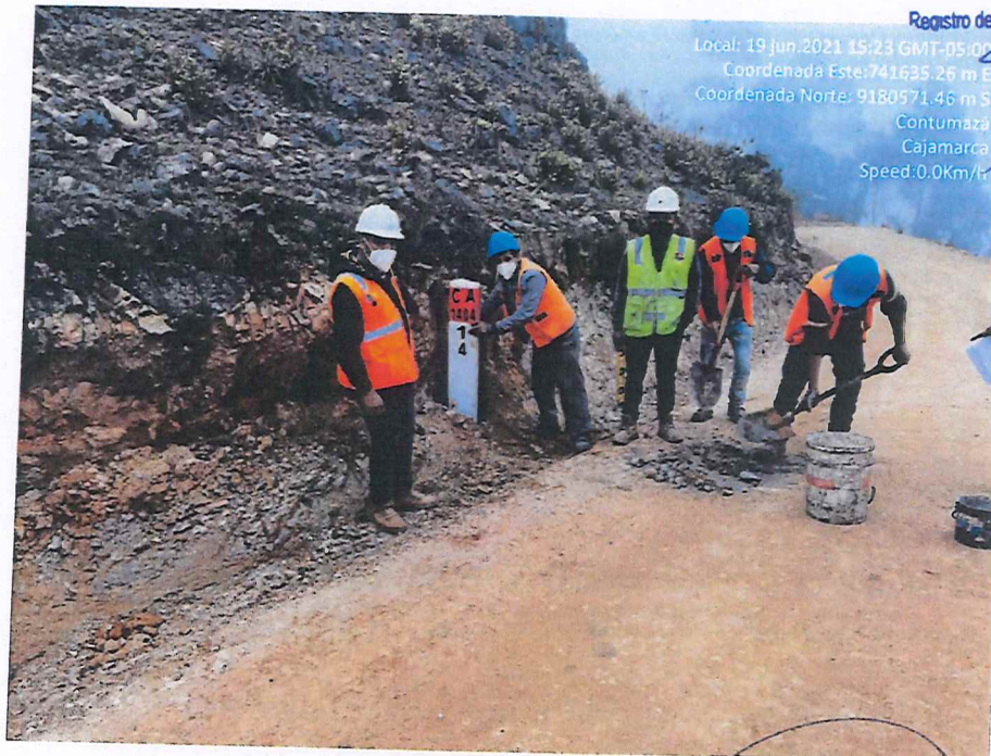
Fotografía 62. Colocación de los postes kilométricos.
