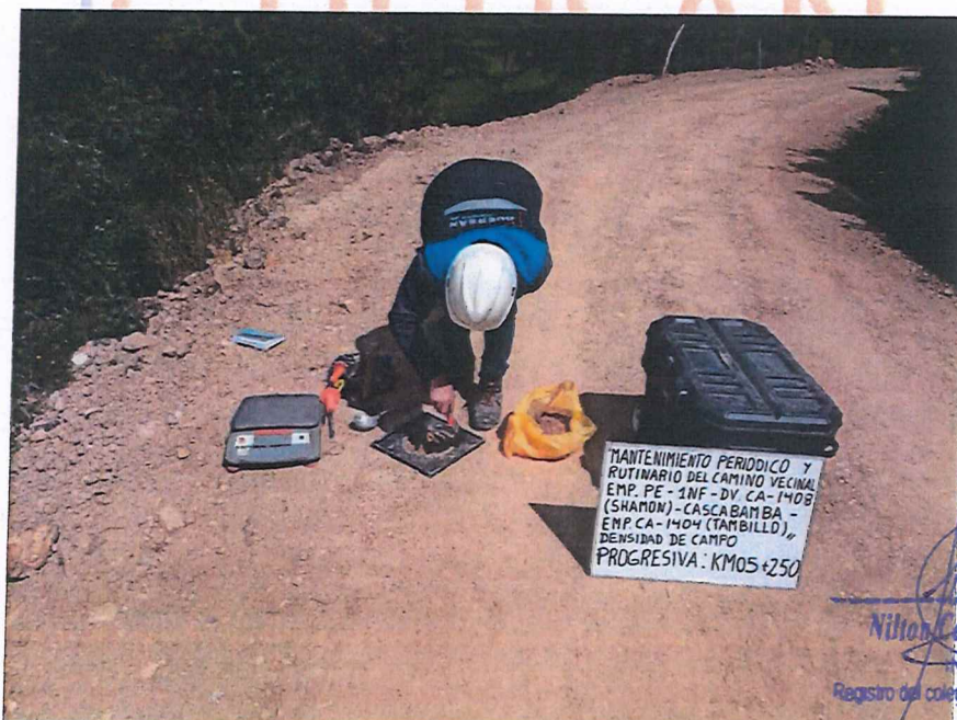
FIGURA N° 22. Ensayo de Densidad de Suelo en Campo. Progresiva 05 +250 (Método del cono de arena).
