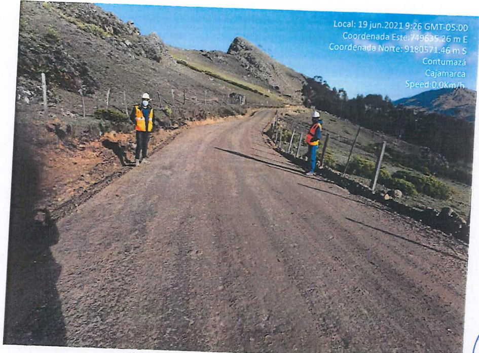
Fotografía 53. Resultado de la compactación del afirmado.
