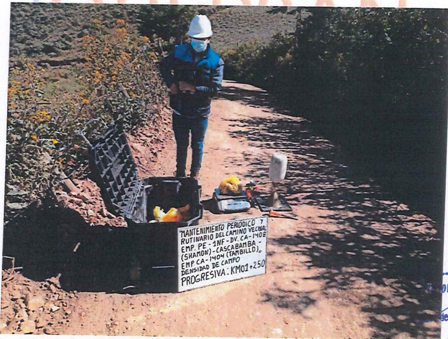
FIGURA N° 6. Ensayo de Densidad de Suelo en Campo. Progresiva 01 + 250 (Método del cono de arena).
